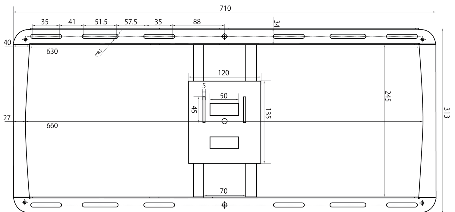
壁面プレート寸法図 寸法は全てミリメートルです
