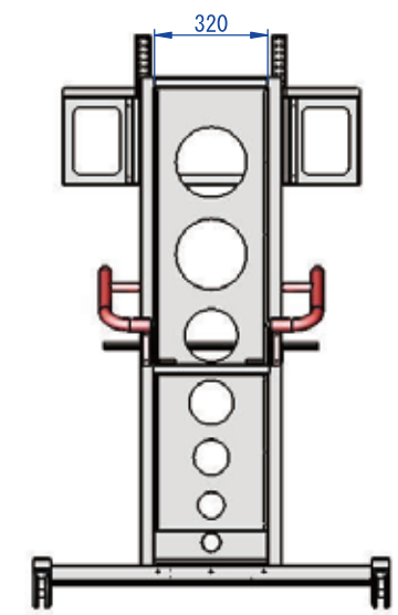
モニター取付金具詳細
