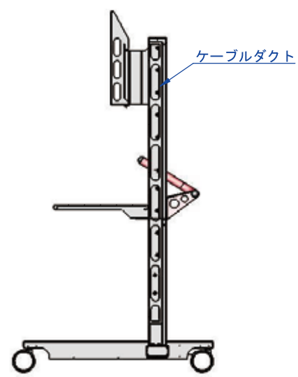
断面図 A-A
