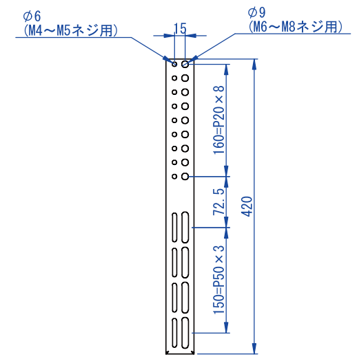
モニター取付金具詳細
