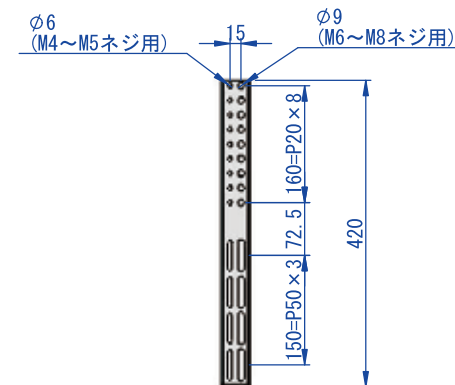
モニター取付金具詳細
