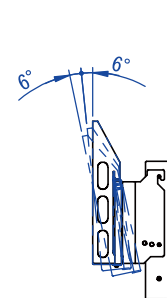
チルト詳細
