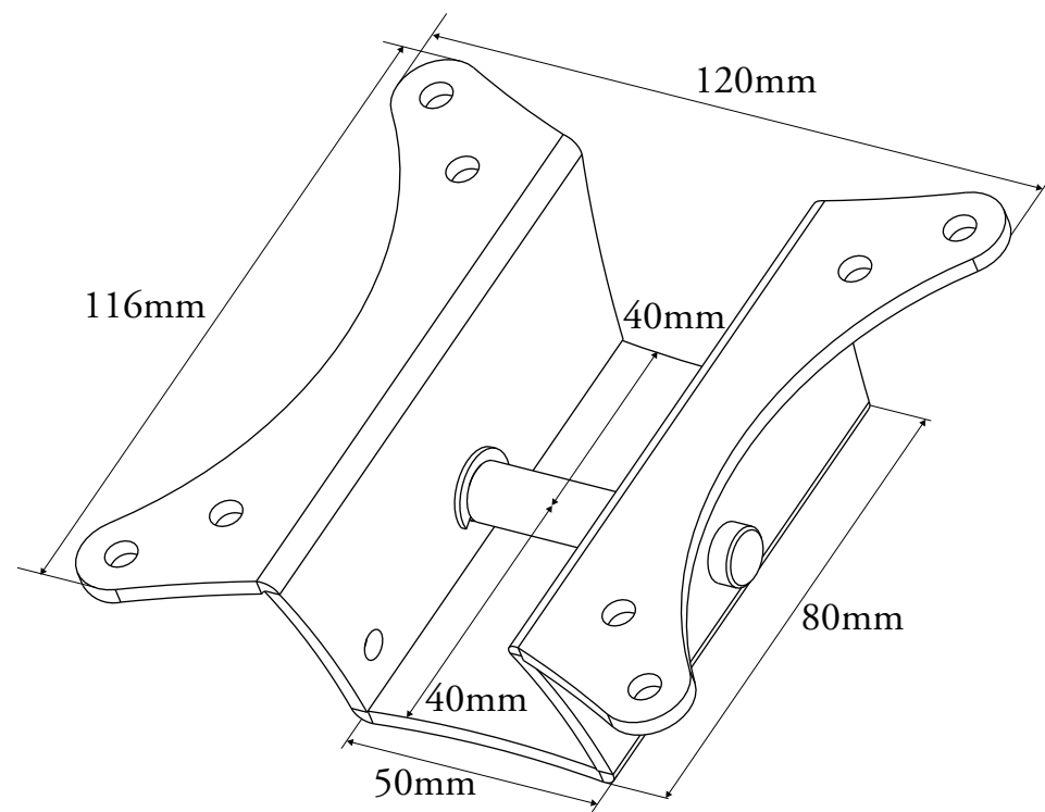
テレビ側プレート
