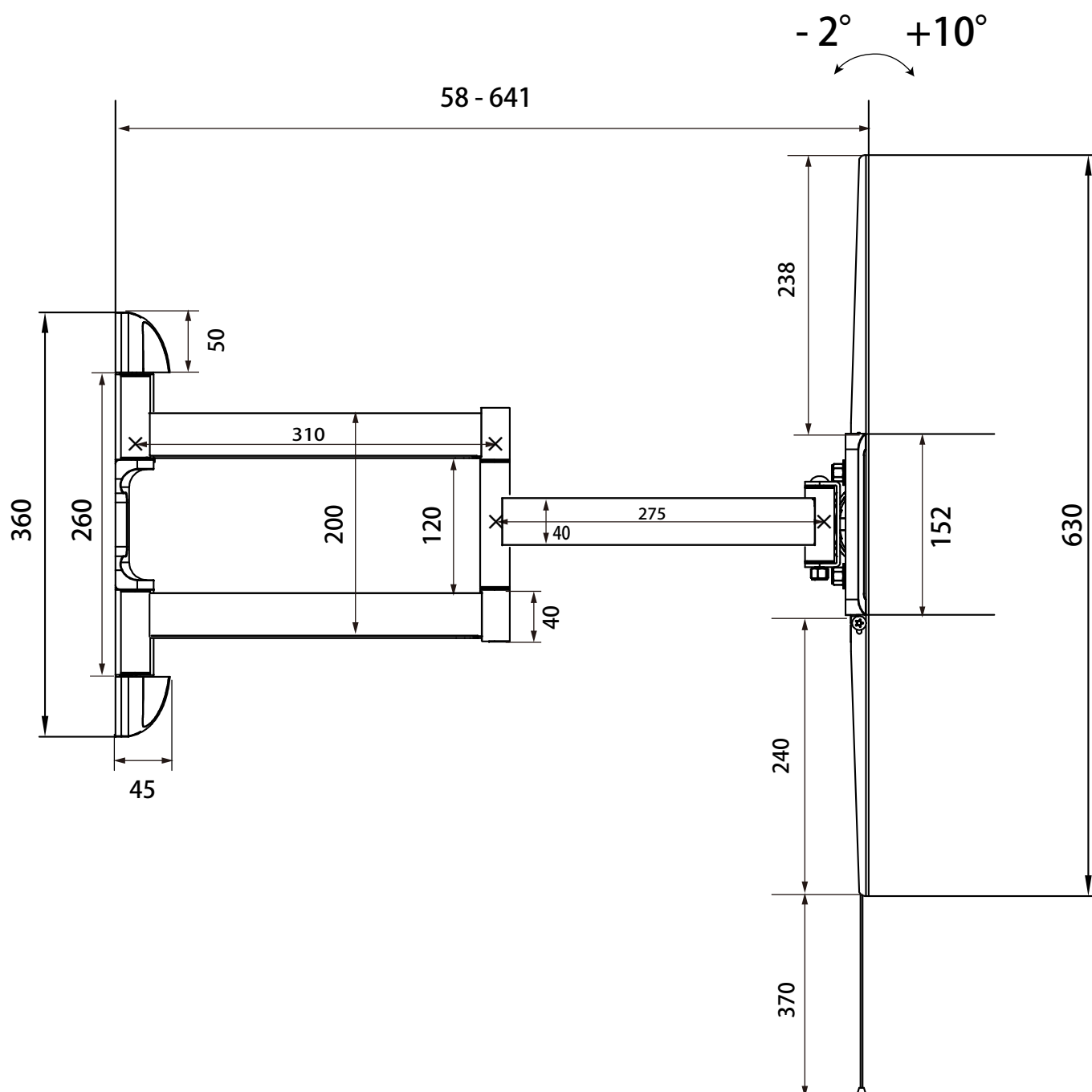
側面図
