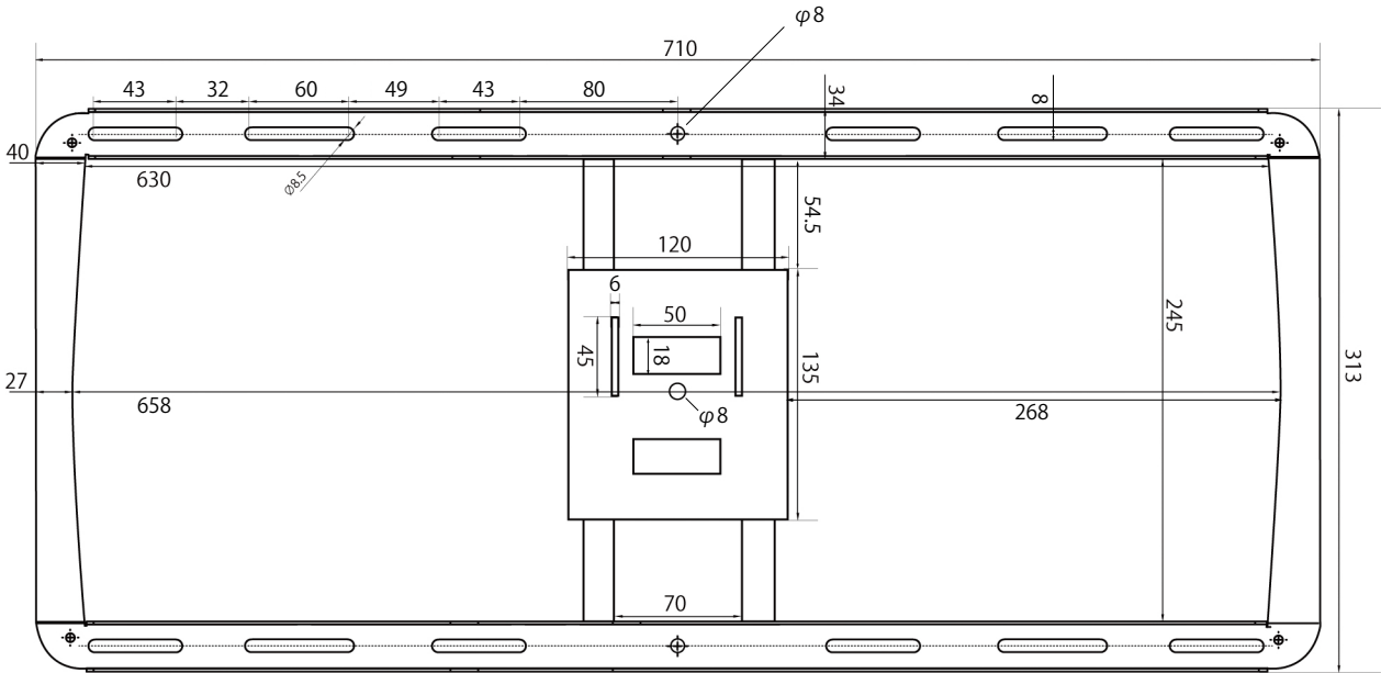
壁面プレート寸法図 寸法は全てミリメートルです
