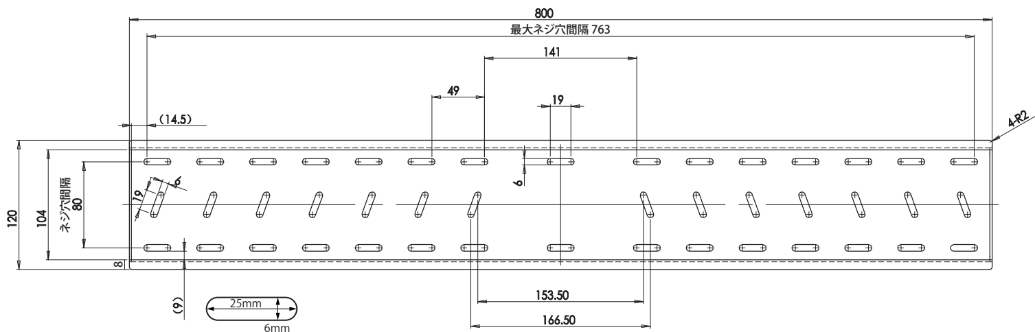
壁側取り付けプレート
