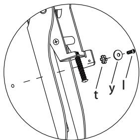
取付け順序
