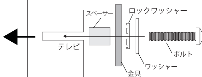
M6/M8 ボルト取付けの場合
