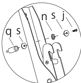
M5 ボルト取付けの場合
