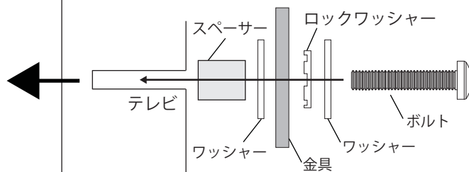
M4/M5 ボルト取付けの場合
